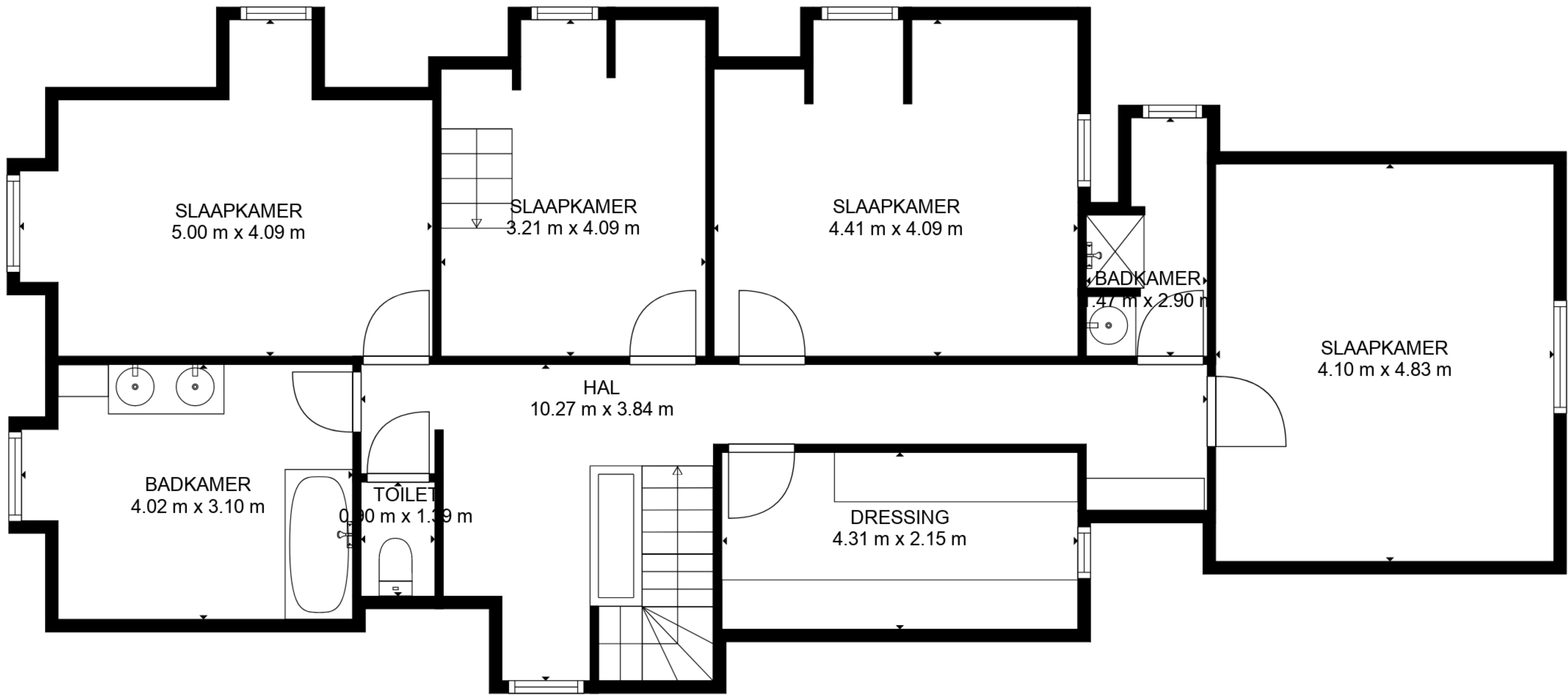
2. VERDIEPING
